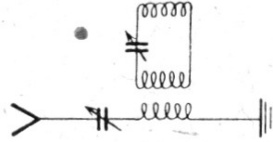
Abb. 460 a bis f. Detektorempfänger.
